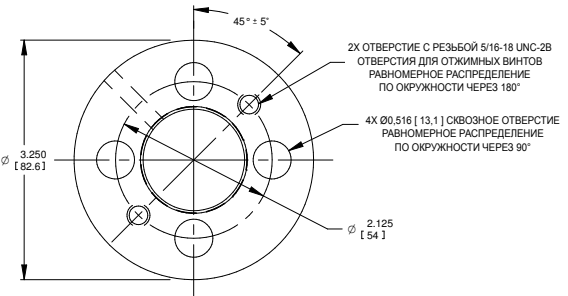
РАЗРЕЗ В-В ФЛАНЕЦ
